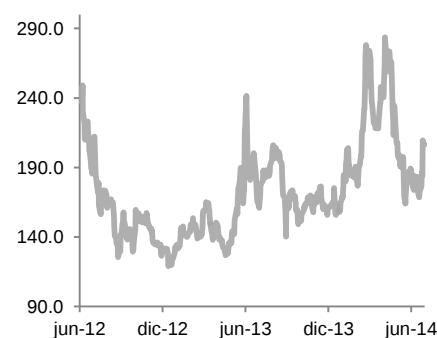
Gráfico 2: CDS, Rusia
