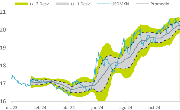
USDMXN
